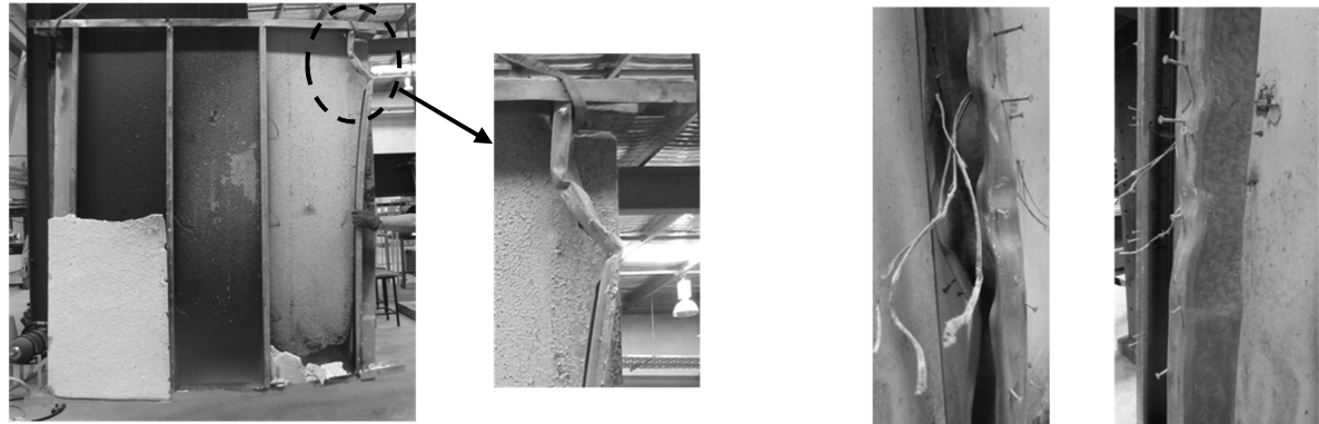
a. T1 – Stud 1
